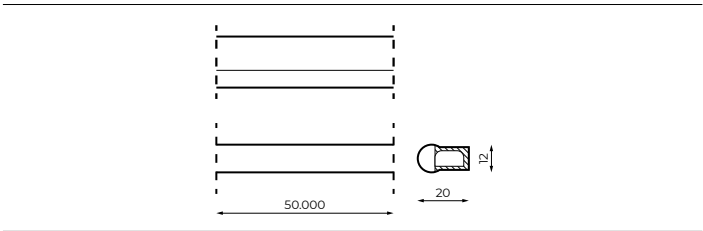
ESQUEMA DE DOBLADO
