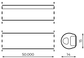
ESQUEMA DE DOBLADO
